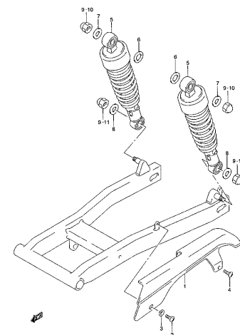
VL250Y 000_047 CHAIN CASE
