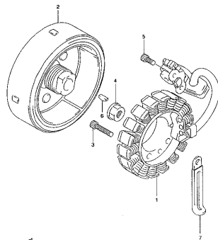
VL250Y 000_019 MAGNETO
