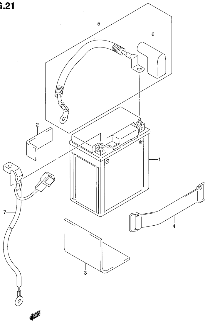
FIG.21 (D-6) バッテリー
