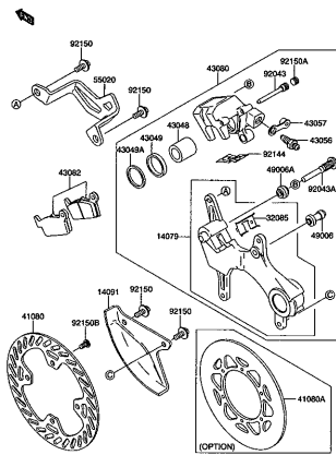
RM-Z250K4 000_037 REAR BRAKE
