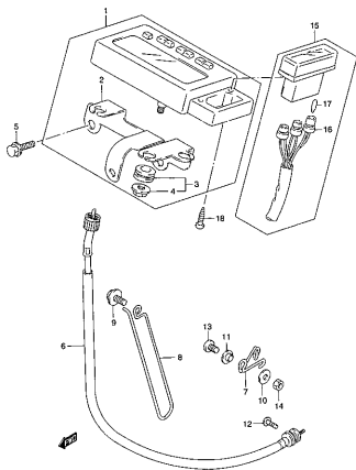
DR250RXKX 000_005 SPEEDOMETER
