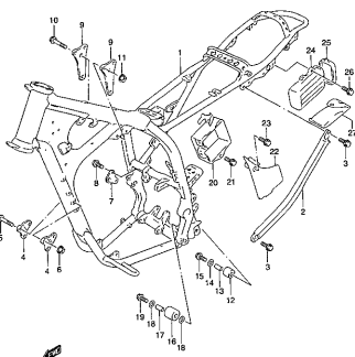
DR250RXKX 000_031 FRAME
