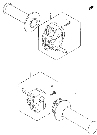
DR250RXKX 000_030 HANDLE SWITCH
