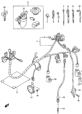
DR250RXKX 000_009 WIRING HARNESS
